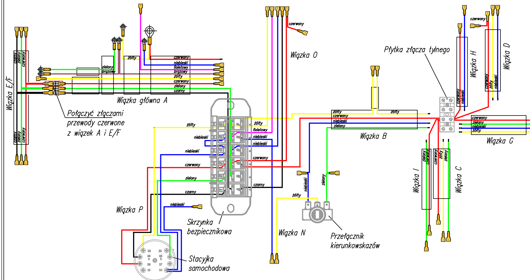
SCHEMAT WIĄZKI
